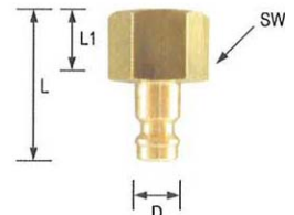
Nippel Innengewinde
