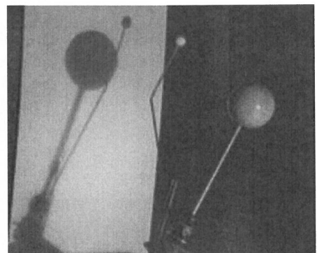
Fig. 17. No eclipse.
