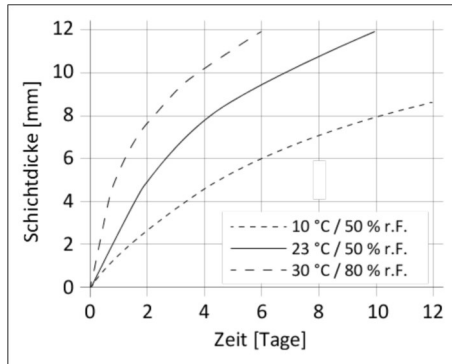
Diagramm 1: Dürchhärtgeschwindigkeit Sikaflex®-252
