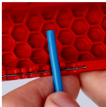
90 22 02 SB : graduation injectée pour un dénudage homogène sur une longueur uniforme, lisible pour les droitiers et les gauchers
