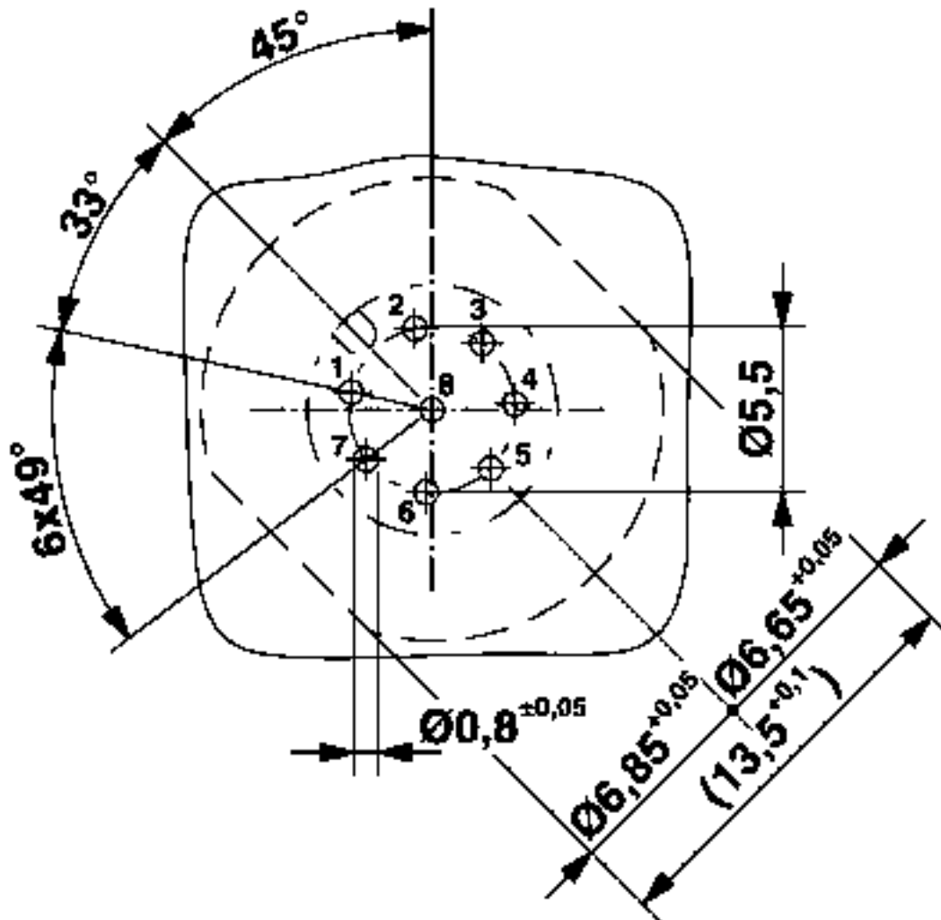
Bohrplan
