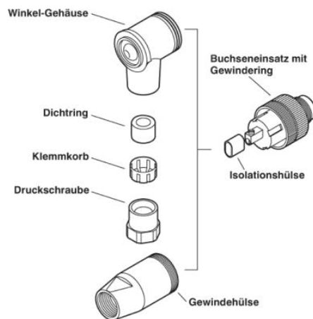
Stecker/Buchse M12
