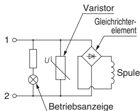
mit Betriebsanzeige/Funkenlöschung
