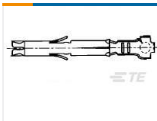
TE Part #170365-3 MINI UNIVERSAL M-N-L SOCKET LP
