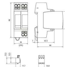
Maßbild DG MP TT 2P 385 FM
