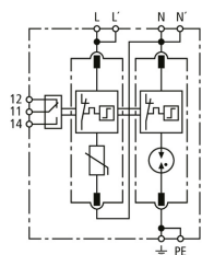
Principalschaltbild DG MP TT 2P 385 FM
