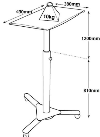
DV- / Dia-Projektionswagen, mit Maßangaben
