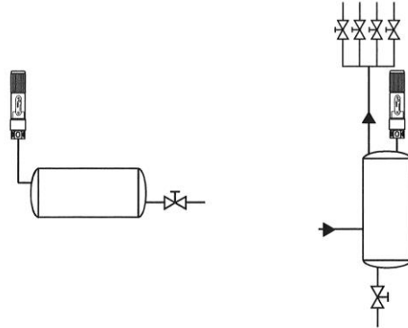
Abb. 1 Beispiel für den standardmäßigen Einbau des Sicherheitsventils
