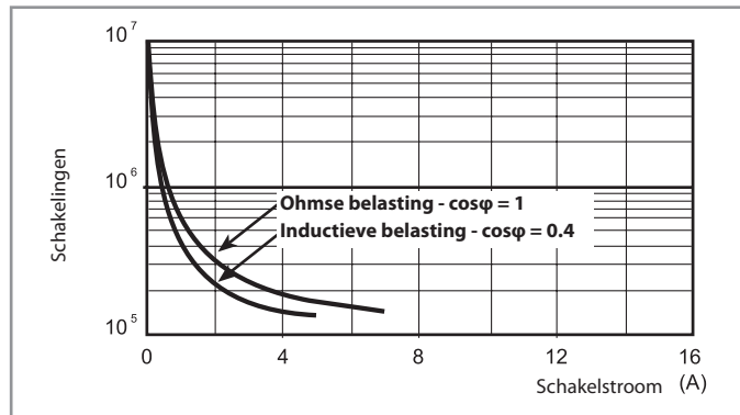
F 55 - Elektrische levensduur bij AC 4 wisselcontacten
