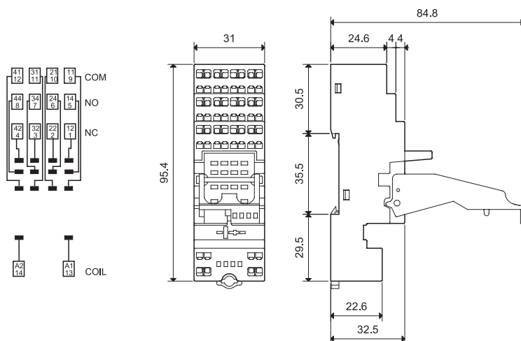
Aansluitvoet + doorverbindstrip
