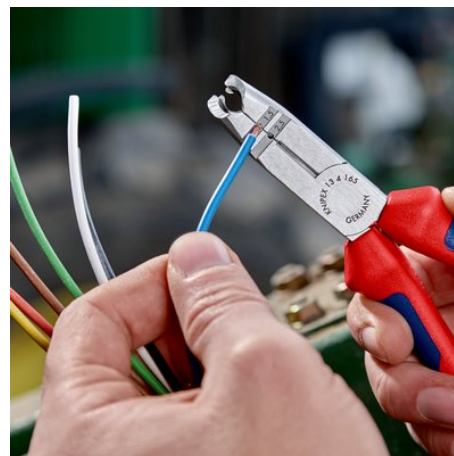
Csupaszító lyukak 1,5 mm 2 és 2,5 mm 2 méretű vezetékhez
