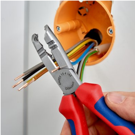
Egyedi vezetők méretre vágása
