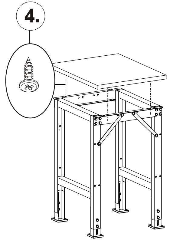
Waagentisch
