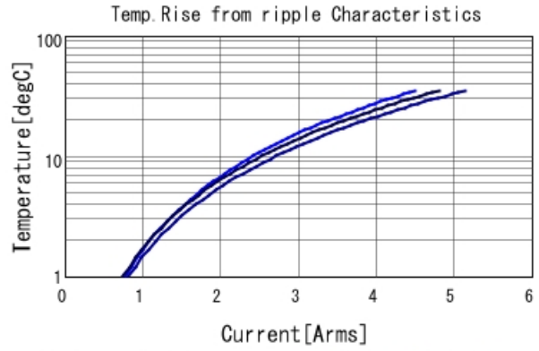
GCJ31CC71E106KA15 Temp. rise ■ 80kHz ■ 400kHz ■ 800kHz
