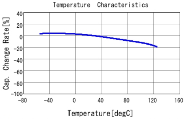
■ GCJ31CC71E106KA15 C-Temp. capchange, DCO. 0V, AC1. 0Vrm
