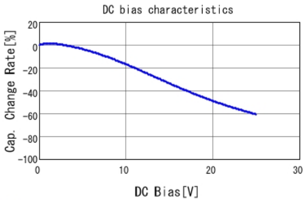
■ GCJ31CC71E106KA15 C-DC bias capchange, 25.0degC, AC1.
