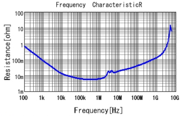
■ GCJ31CC71E106KA15 R DC0V, 25degC
