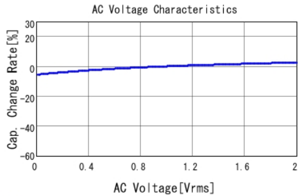
■ GCJ31CC71E106KA15 C-AC Voltage capchange, DC0V, 25.0d
