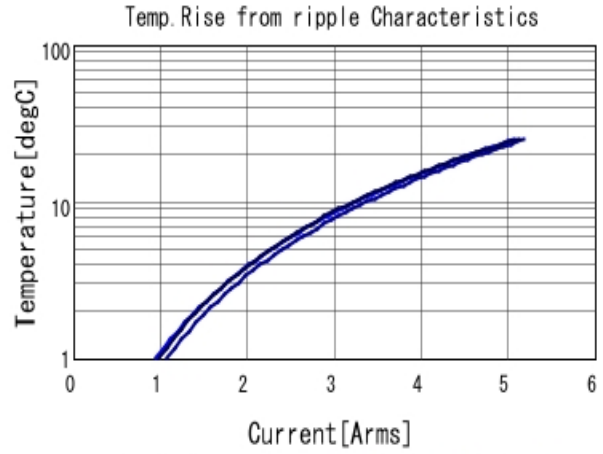
KCM55WR71H336MH01 Temp. rise ■ 50kHz ■ 100kHz ■ 300kHz
