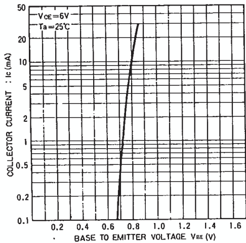
Fig.1 エミッタ接地伝達静特性
