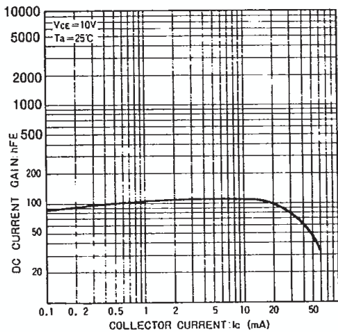
Fig.3 直流電流増幅率—コレクタ電流特性
