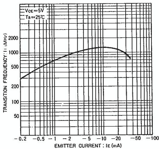
Fig.5 利得帯域幅積—エミッタ電流特性
