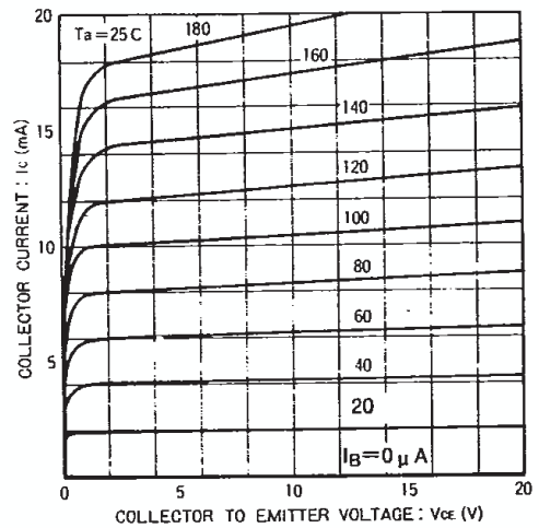
Fig.2 エミッタ接地出力静特性
