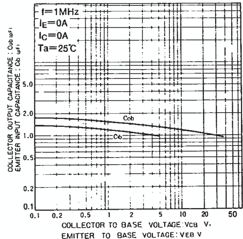
Fig.6 入出力容量—ベース電圧特性
