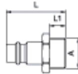
Nippel Außengewinde
