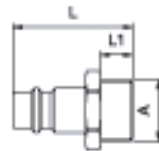
Nippel Außengewinde
