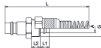
Nippel für Schlauch mit Überwurfmutter, Knickschutzfeder
