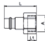
Nippel Innengewinde
