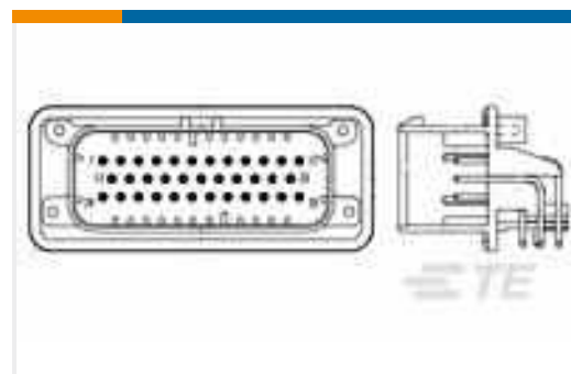
TE Teilnr.:1-776163-1 35POS, PIN DIA 1.3, HDR ASSY, 90DEG, COD 1
