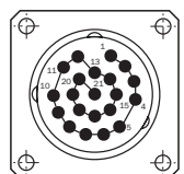
Ansicht Gerätestecker M23, 21-polig am Encoder, Parallel
