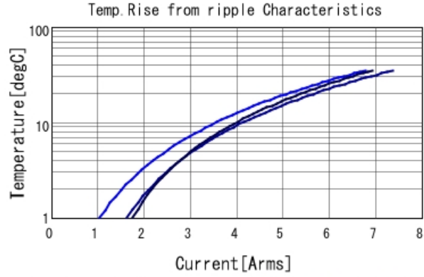
GCM32EC71A476KE02 Temp. rise ■ 60kHz ■ 300kHz ■ 600kHz
