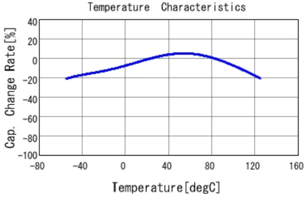
GCM32EC71A476KE02 C-Temp. capchange, DCO. 0V, ACO. 25Vr
