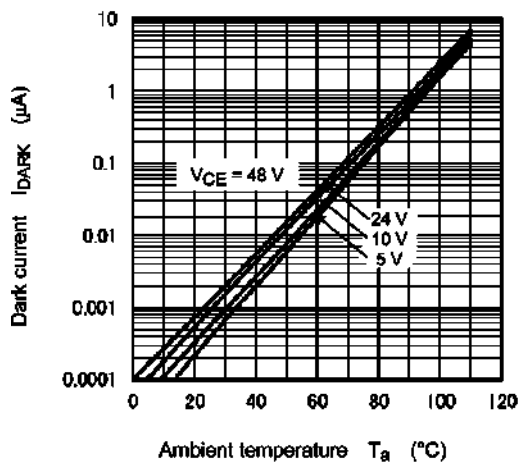
Fig. 11.11 I_{\text{DARK}} - T_a
