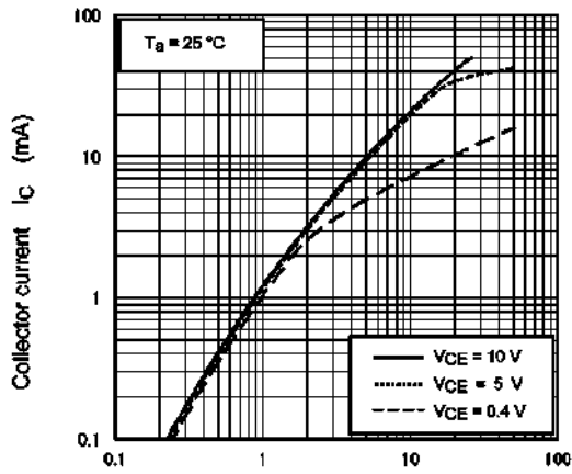
Fig. 11.9 I_C - I_F
