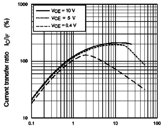
Fig. 11.10 I_C/I_F - I_F
