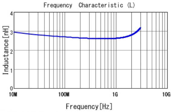
■ LQG15HN2N7C02 L
