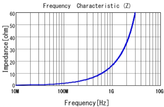
■ LQG15HN2N7C02 |Z|
