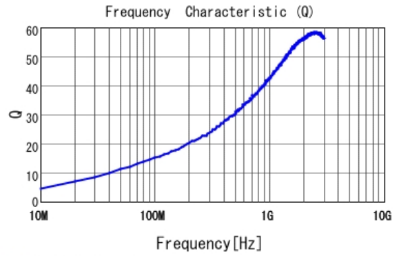
■ LQG15HN2N7C02 Q
