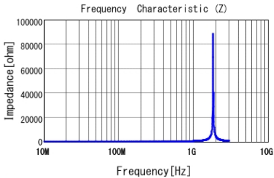
■ LQW2BAS68NJ00 |Z|
