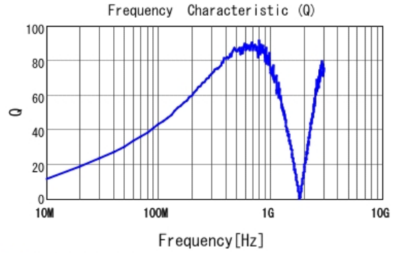
■ LQW2BAS68NJ00 Q
