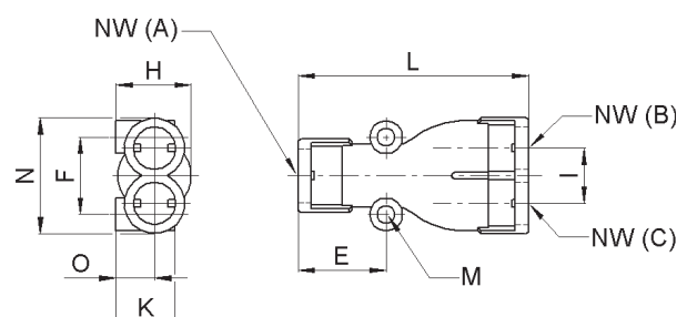
Dimensions Dimensionen
