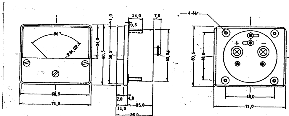
Typ ST-670 cl. 2,5 (Grösse 71x60,5mm)
