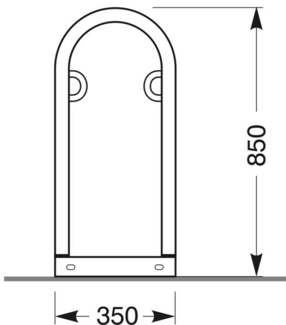
Technische Ansicht: Maße Anlehnbügel -Track- (Art. track31)
