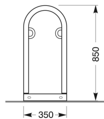
Modellbeispiel: Reihenanlehnbügel -Track- (3er) aus Stahl, mit 6 Einstellplätzen (Art. Track33)
