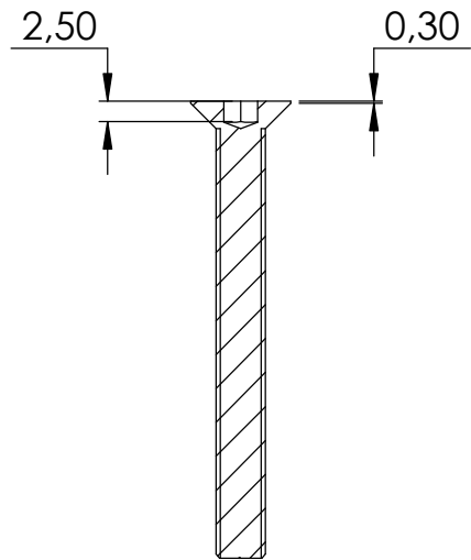
SCHNITT A-A
