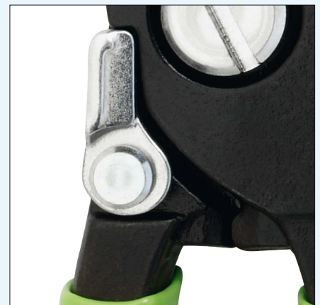
mit Öffnungsfeder und Sicherheitsverschluss with opening spring and lock
