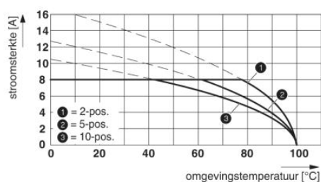
Deratingcurve voor: TFMC 1,5/...-ST-3,5 met MCV 1,5/...-G-3,5
