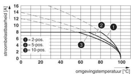
Type: TFMC 1,5/...-ST-3,5 met MC 1,5/...-G-3,5
