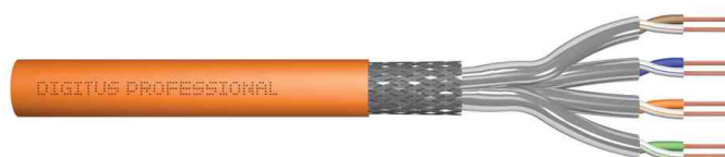
Câble d'installation cat. 7, S/FTP, PiMF, duplex
