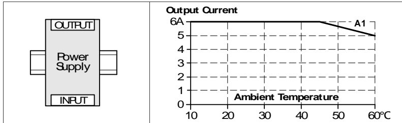
Bild 22-3 Einbaulage A (Standard- Einbaulage)
