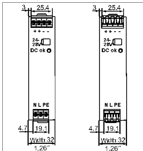
Bild 20-1 Frontansicht CS5.241, CS5.241-C1 CS5.241-S1
