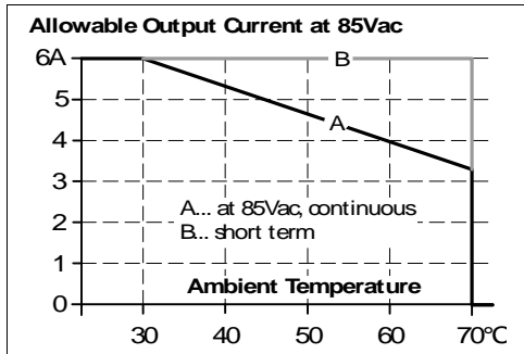
Bild 3-5 Eingangsspannungsderating
