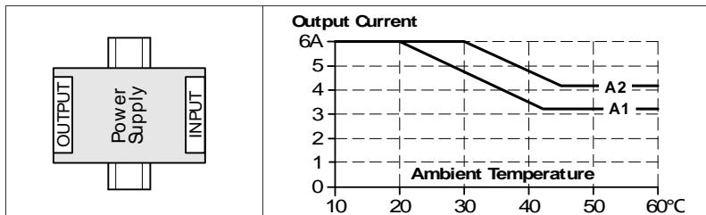
Bild 22-7 Einbaulage E (Horizontal gegen den Uhrzeigersinn)
