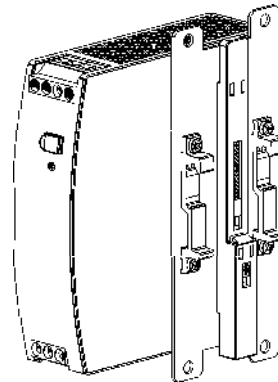
Seitliche Montage ohne DIN-Schienen-Halterungen
