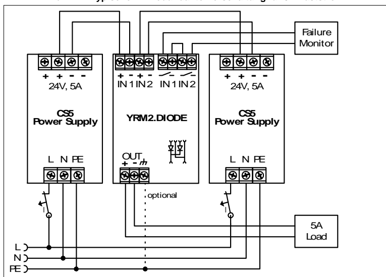
Bild 21-1 Typische 1+1 redundante Verschaltung für 5A Laststrom
