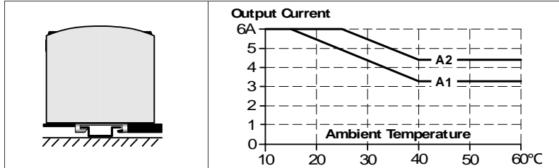
Bild 22-5 Einbaulage C (Tischmontage)
