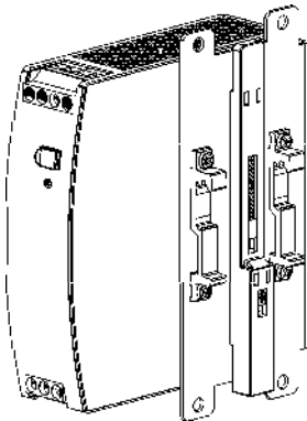
Seitliche Montage mit DIN-Schienen-Halterungen
