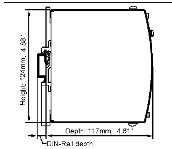
Bild 20-2 Seitenansicht
