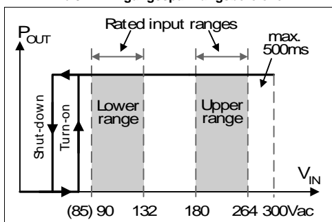
Bild 3-1 Eingangsspannungsbereiche
