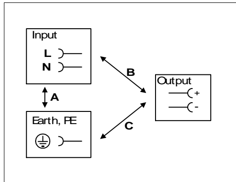
Bild 17-1 Spannungsfestigkeit
