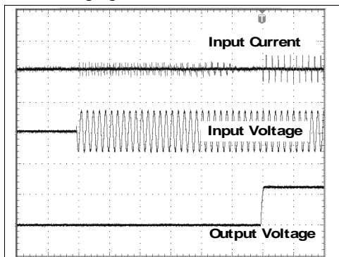
Bild 5-1 Typisches Eingangseinschaltstromverhalten
