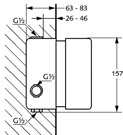
Maßzeichnung II
