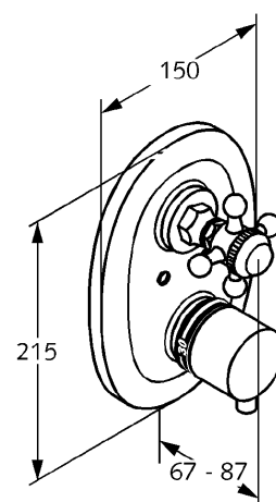
Maßzeichnung I
