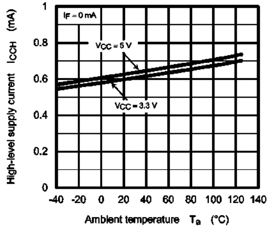
Fig. 12.2.8 I_{CCH} - T_a
