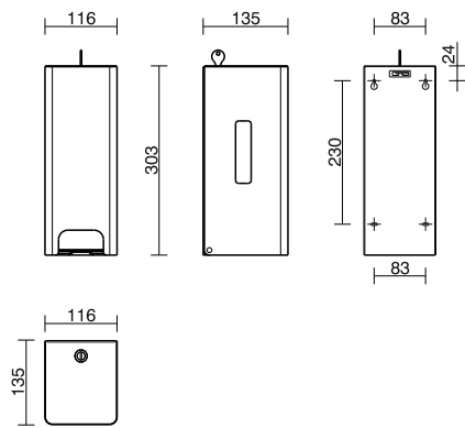
706700 Toilettenpapierspender für 2 Rollen
