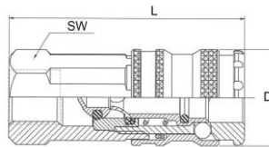
Innengewinde
