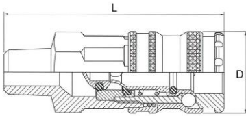
Außengewinde
