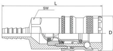
Schlauchanschluss
