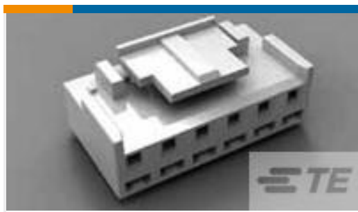
TE Teilnr.:1-1123722-3 3.96 EP PLUG HSG 3P(NATURAL)
