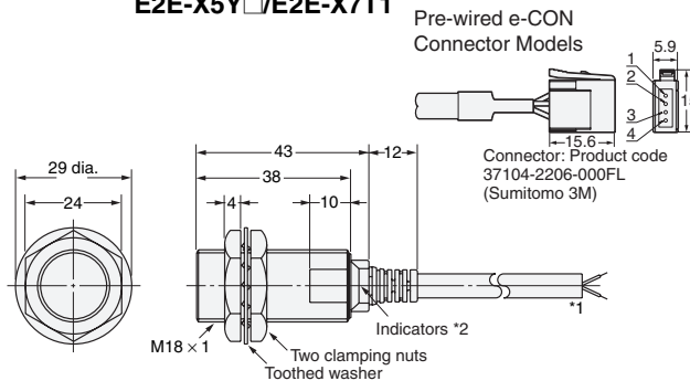
Diagram 14 E2E-X7D□/E2E-X5E□/F□ E2E-X5Y□/E2E-X7T1
