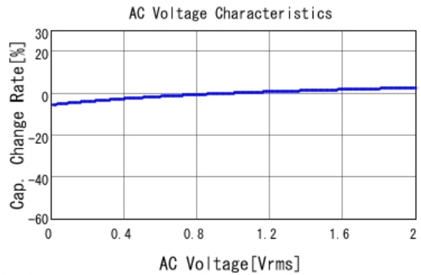
■ GCJ31CC71E106KA15 C-AC Voltage capchange, DC0V, 25.0d
