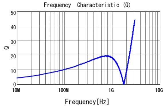
■ LQG15HH39NJ02 Q
