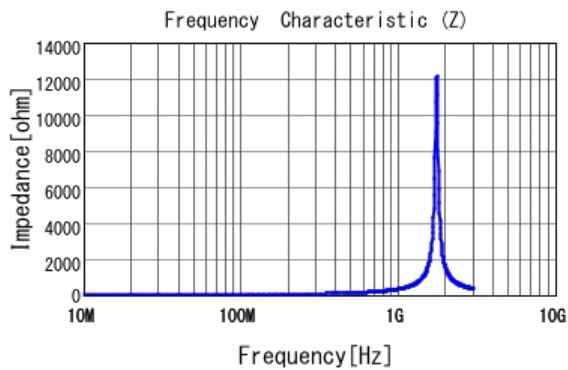
■ LQG15HH39NJ02 |Z|
