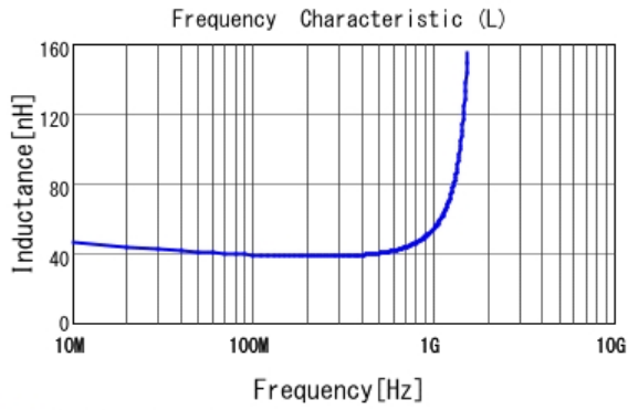
■ LQG15HH39NJ02 L
