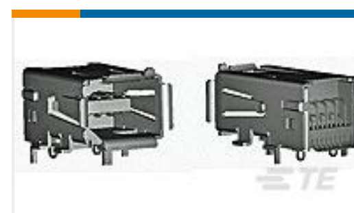
TE Part #2069552-1 INDUSTRIAL MINI I/O HDR ASSY E
