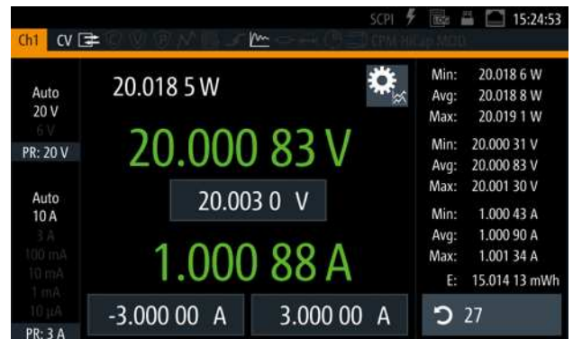
Quellbetrieb
