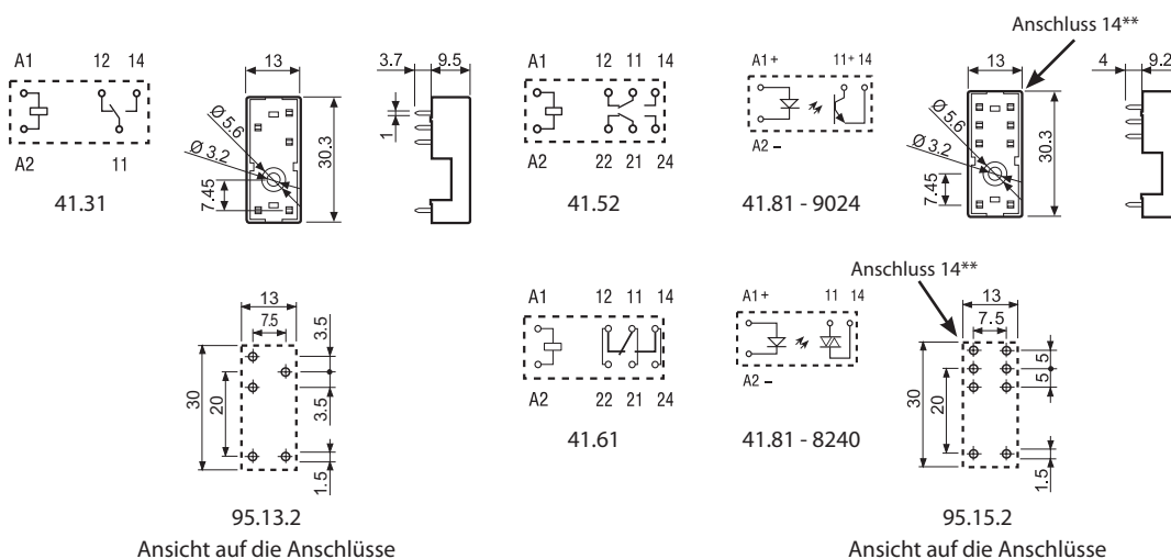
Ansicht auf die Anschlüsse
