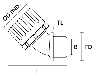
HeliaGuard Verschraubung, 45° mit starrem Außengewinde
