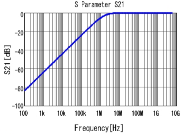
■ GCM155L81H102KA37 S21 DCOV, 25degC
