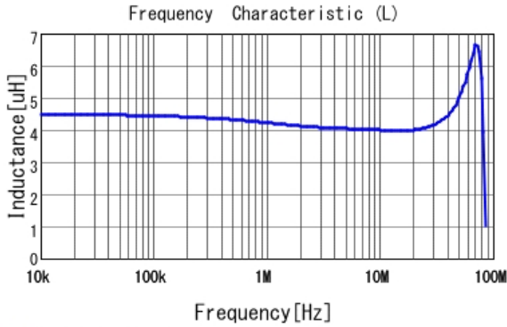
■ 1227AS-H-4R7M L
