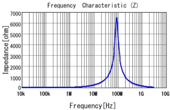
■ 1227AS-H-4R7M |Z|
