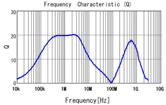
■ 1227AS-H-4R7M Q
