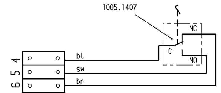
Schaltbild
