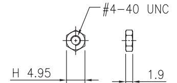
NUT *2PCS
