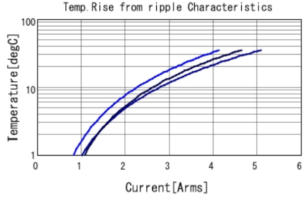
GRJ31CR71H475KE11 Temp. rise ■ 100kHz ■ 500kHz ■ 1MHz
