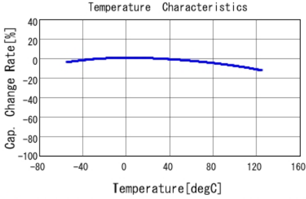
■ GRJ31CR71H475KE11 C-Temp. capchange, DCO. 0V, ACO. 1Vrm
