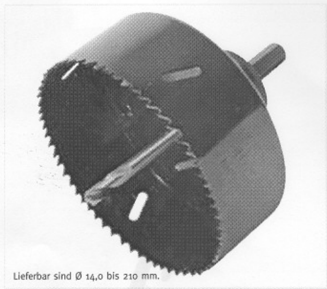
Combi-Verzahnung 4/6 ZpZ
